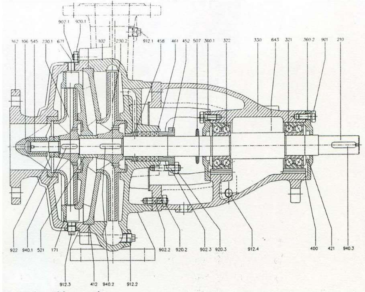
Πίνακας Ανταλλακτικών
