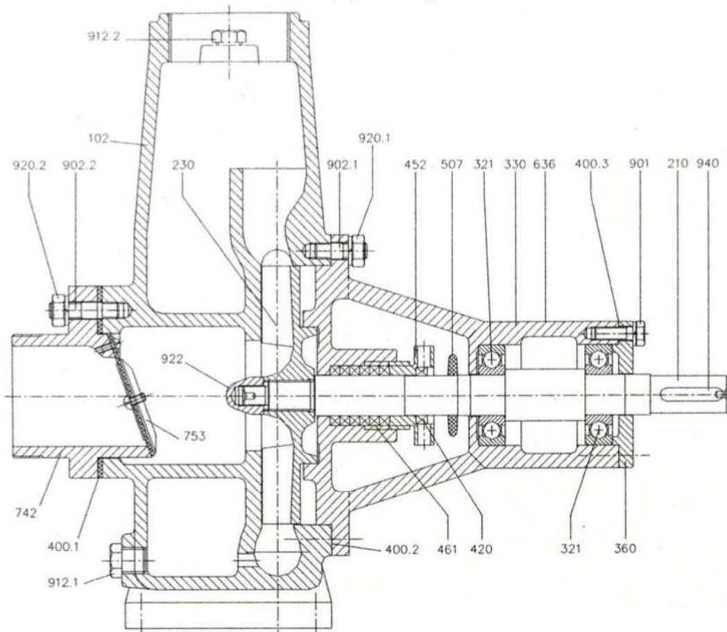
Πίνακας Ανταλλακτικών
